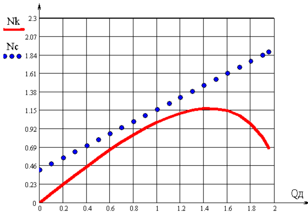
Рисунок 7 — Розрахункові характеристики корисної N_k та спожитої N_c потужності насоса НМ-2500-230
