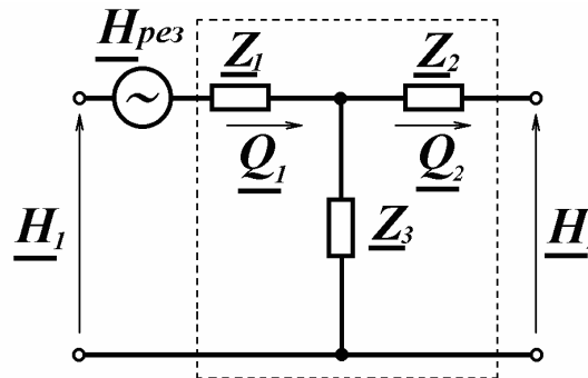
Рисунок 4 — Пасивний чотириполосник
