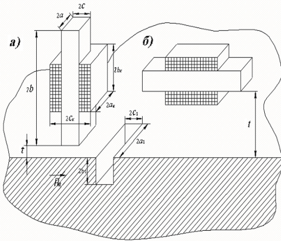
Рисунок 1 – Геометрическая модель системы феррозонд–дефект
