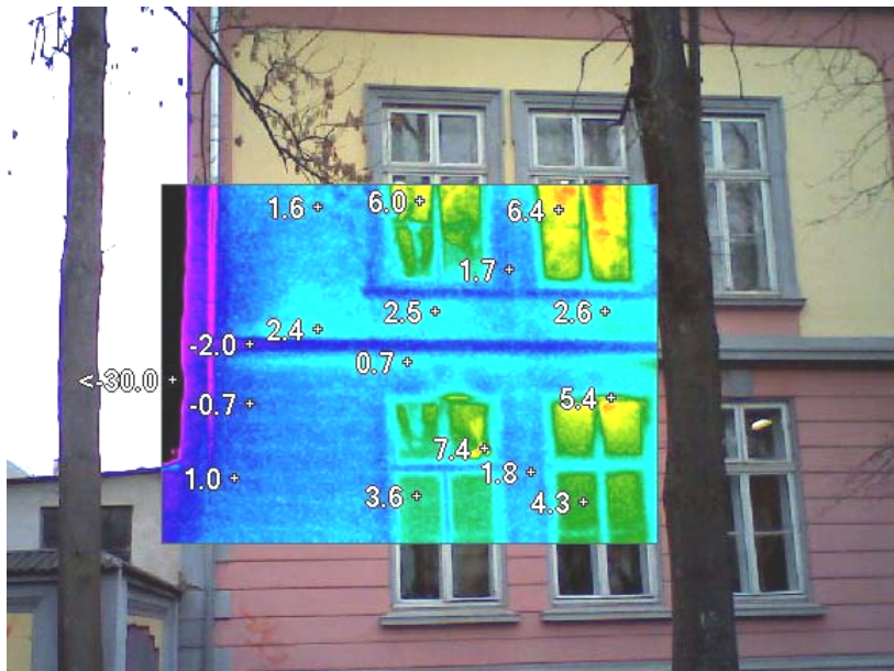
Рисунок 3 – Тепловізійне зображення зовнішньої стіни будівлі
