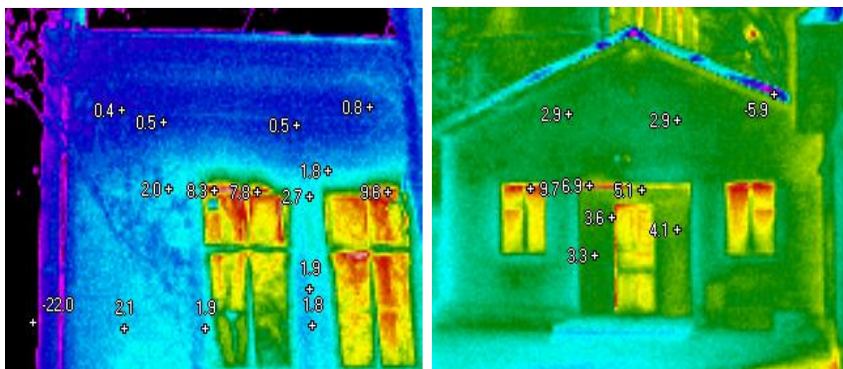
Рисунок 2 – Тепловізійні зображення досліджуваної будівлі
