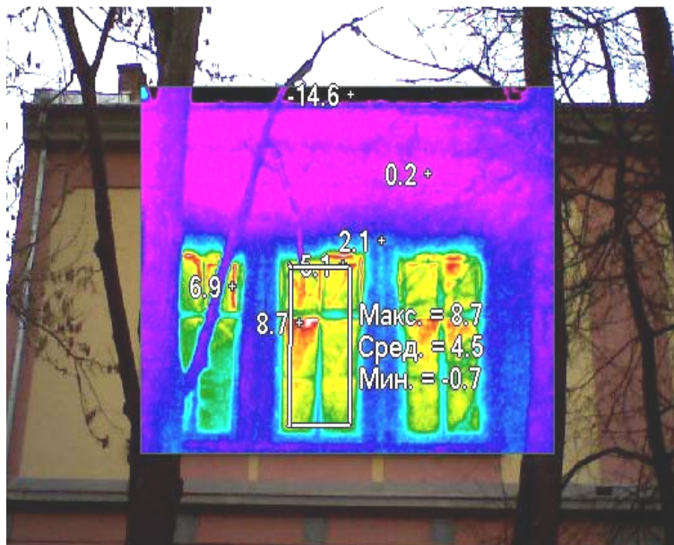
Рисунок 7 – Визначення середнього значення температури поверхні віконних проїомів
