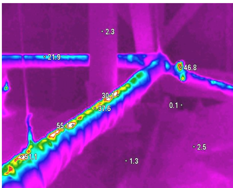
Рисунок 8 – Місця витоків тепла у системі опалювання
