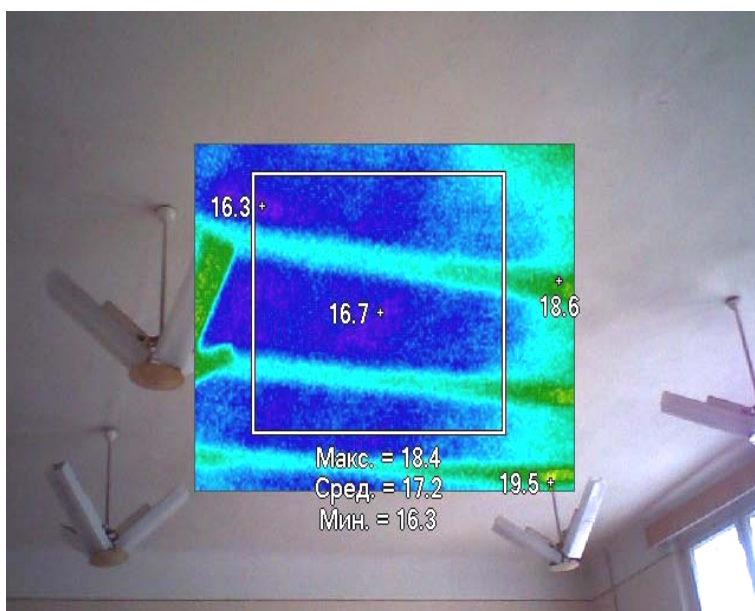
Рисунок 6 – Визначення середнього значення температури поверхні перекриття горища
