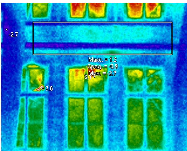
Рисунок 5 – Визначення середнього значення температури поверхні зовнішніх стін
