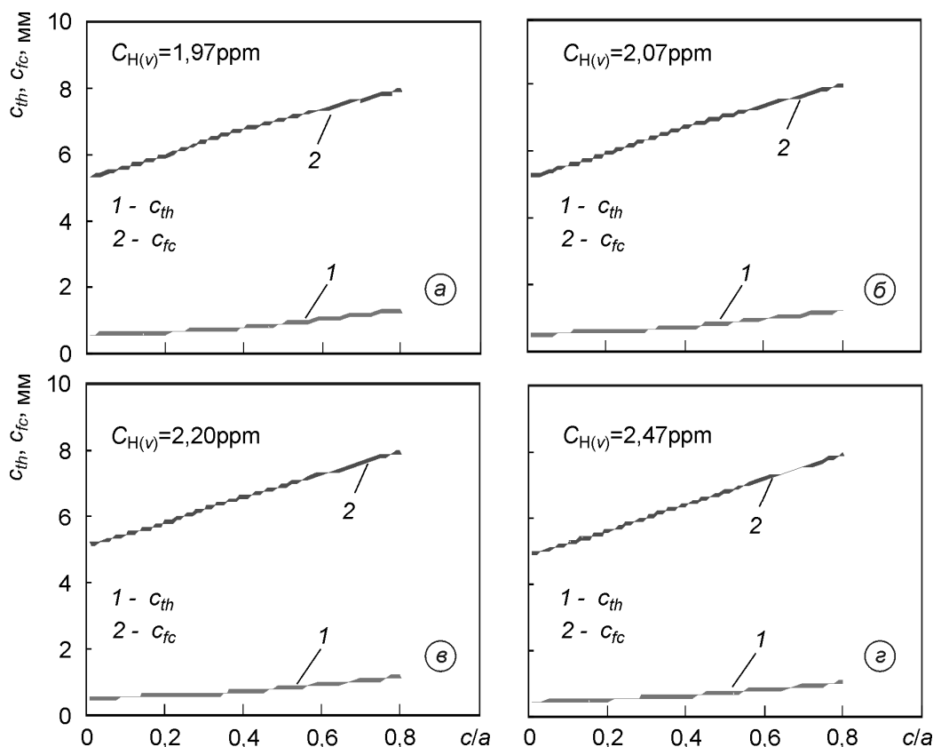
Рисунок 10 – Діаграми критичних розмірів дефектів c_{th} та c_{fc} у трубопроводі 526 × 50 мм за різних концентрацій водню в об’ємі металу
