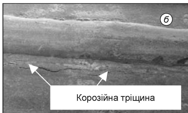
Рисунок 1 – Дефекти типу „повздожжні риси” на поверхні труби, які знаходяться поблизу повздожжніх зварних швів (а) та ініційовані ними корозійне розтріскування двошовної зварної труби зі сталі Х70 (б) [6]
