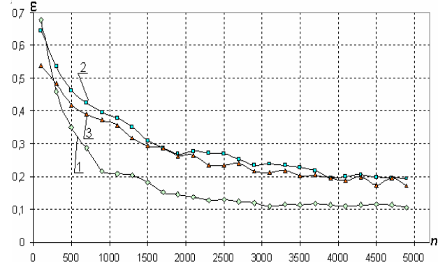
1 – витрата 3 \text{ м}^3/\text{год.} ; 2 – витрата 5 \text{ м}^3/\text{год.} ; 3 – витрата 8 \text{ м}^3/\text{год.}
