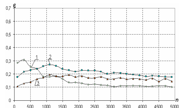
1 – витрата 3 \text{ м}^3/\text{год.} ; 2 – витрата 5 \text{ м}^3/\text{год.} ; 3 – витрата 8 \text{ м}^3/\text{год.}
