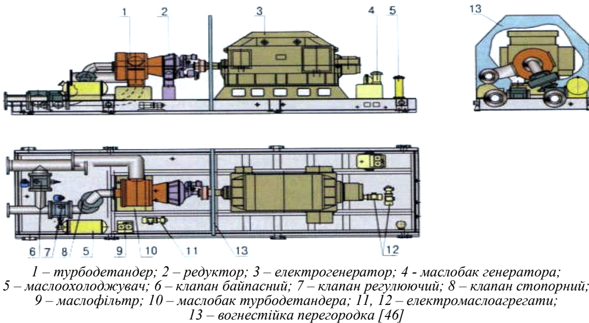
Рисунок 5 – Схема комплектування установки ДГА-2500СД1
