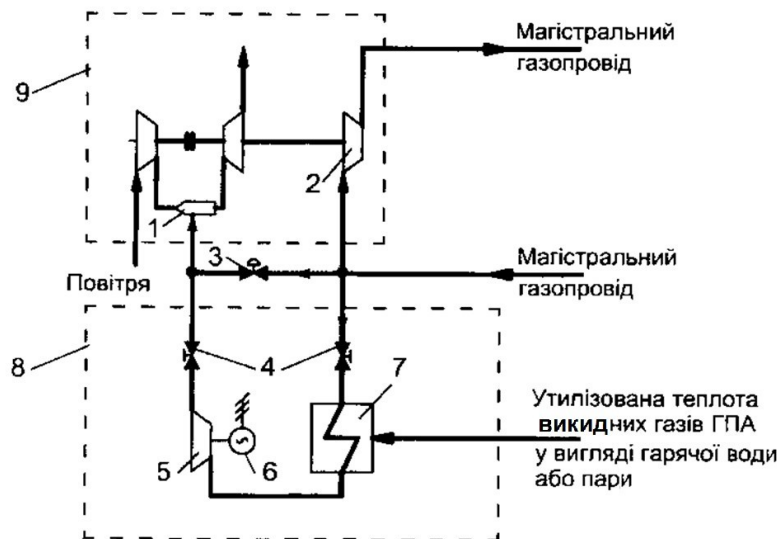
1 - камера згоряння ГТУ; 2 - нагнітач природного газу; 3 - вузол редукування; 4 - крани; 5 - турбодетандер; 6 - електрогенератор; 7 - підігрівник газу; 8 - УТДУ; 9 - газотурбінний агрегат Рисунок 2 – Принципова схема УТДУ для вироблення електроенергії на КС
