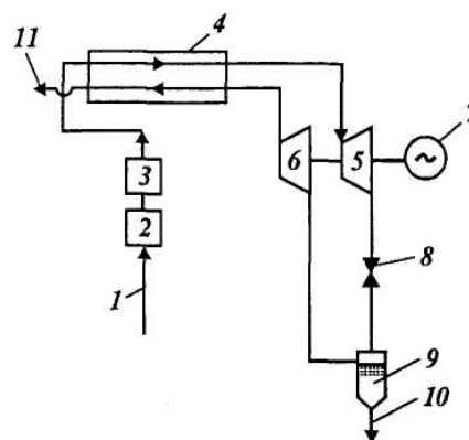
1 - підведення газу до ГРС; 2 - установка осушування газу; 3 - установка очищення газу; 4 - теплообмінник; 5 - турбодетандер; 6 - дотискувальний компресор; 7 - електрогенератор; 8 - дросель; 9 - сепаратор; 10 - відвід зрідженого метану; 11 - відвід газу споживачу
