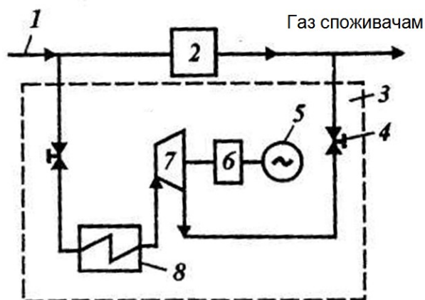
1 – підведення газу до ГРС; 2 – ГРС (ГРП); 3 – УТДУ; 4 – кран; 5 – електрогенератор; 6 – редуктор; 7 – турбодетандер; 8 – підігривач газу
