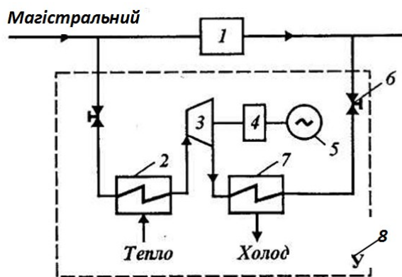
1 - ГРС (ГРП); 2 - підігрівник газу; 3 - турбодетандер; 4 - редуктор; 5 - електрогенератор; 6 - кран; 7 - споживач холоду; 8 - УТДУ
