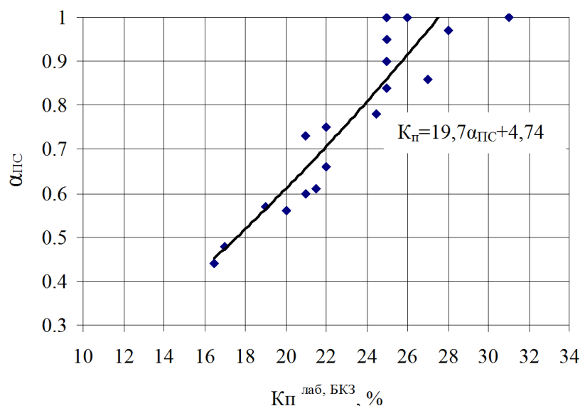
Рисунок 4 – Залежність \alpha_{ПС}=f(K_n) для нижньосарматських відкладів Хідновицького родовища
