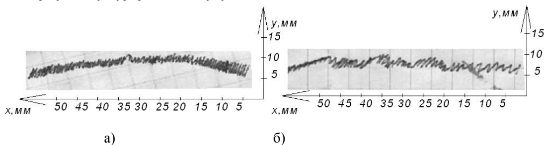
Рисунок 2 – Графічна реєстрація кривих траєкторій переміщення точок віброрами бурового вібростата ЛВС -5 над передньою лівою пружинною віброопорою: а – при незавантаженому ситополотні; б – при наявності промивальної рідини на ситополотні.
