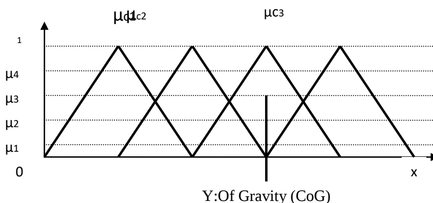
Рисунок 2.7 – Метод дефазифікації як перетворення нечіткого результату виведення у чіткий вихід на основі методу центру тяжіння (CoG)
